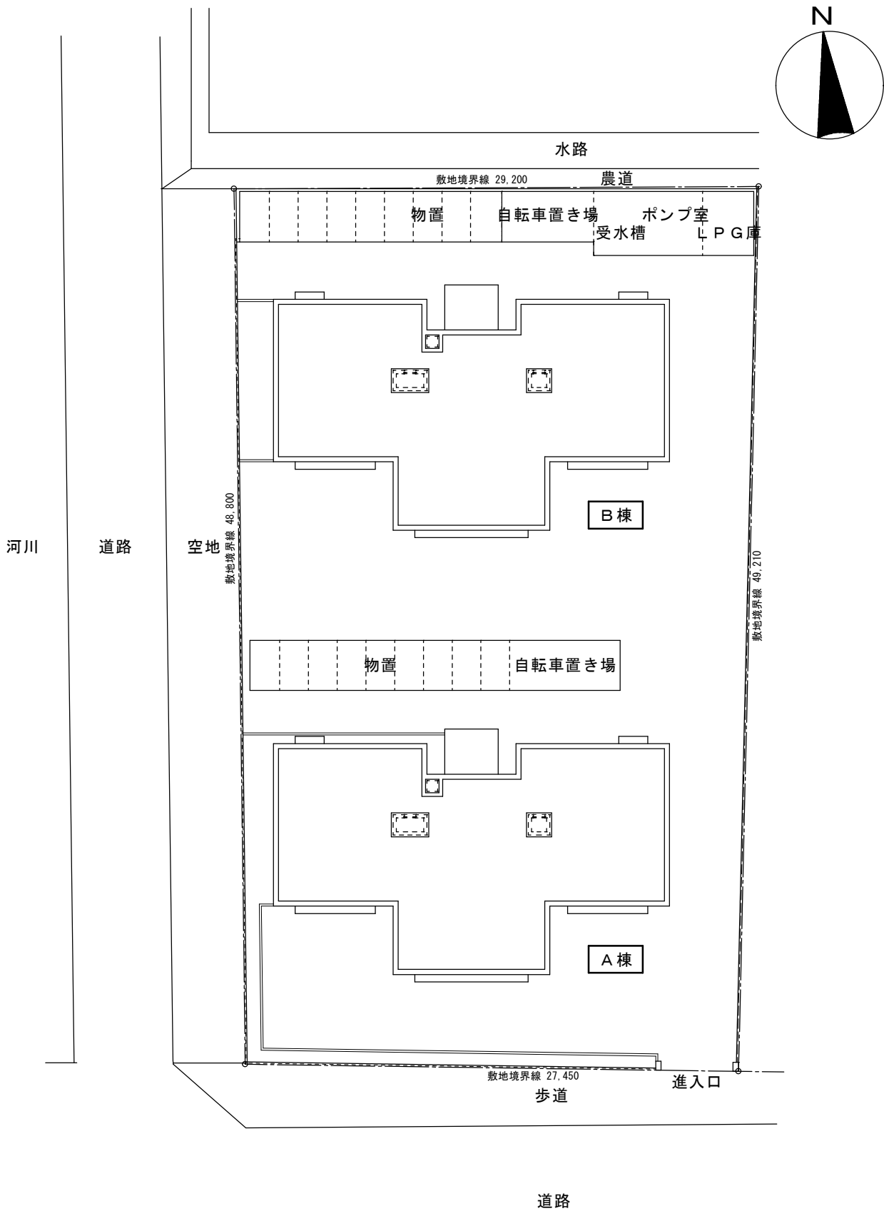
詰田川待機宿舎配置図
