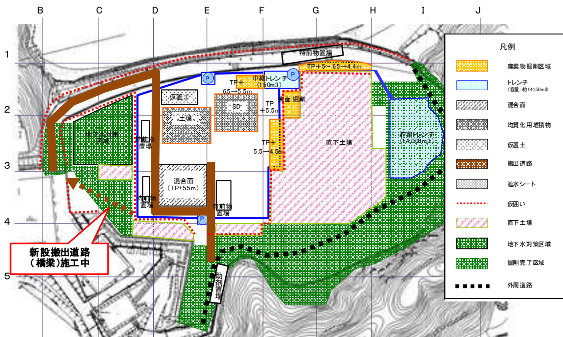
図2 平成27年7月掘削計画
