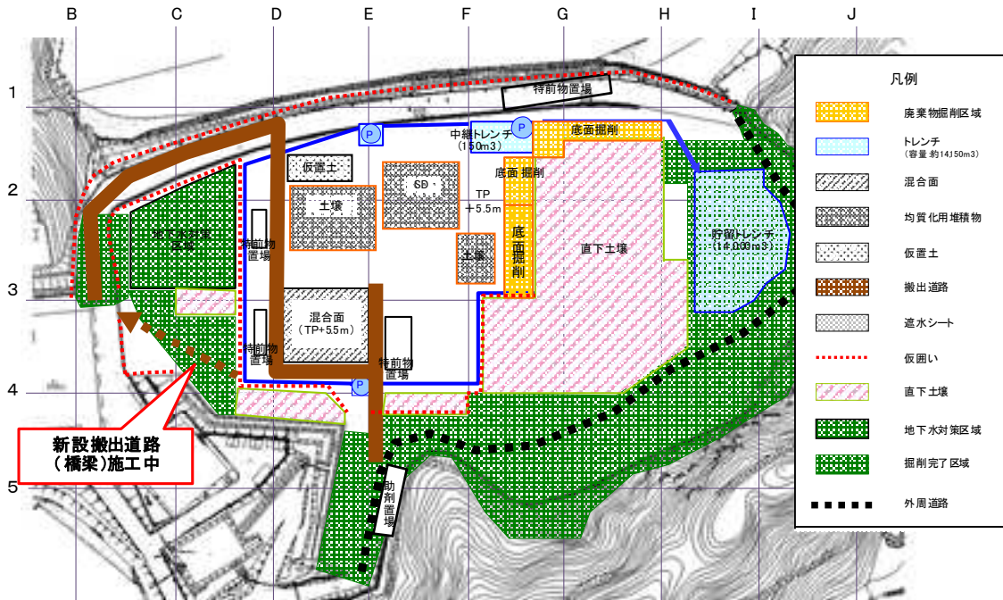
図1 平成27年6月掘削実績
