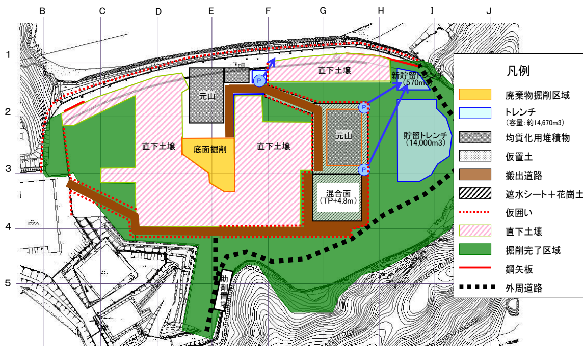
図2 平成28年10月掘削計画
