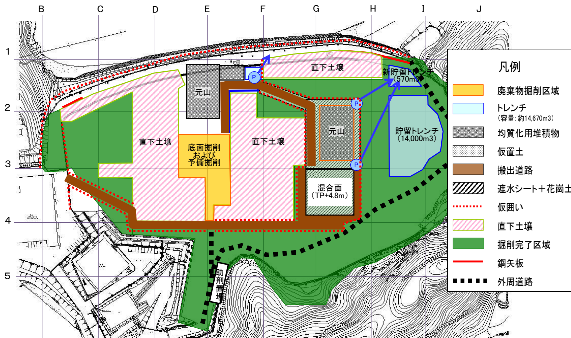
図1 平成28年9月掘削実績
