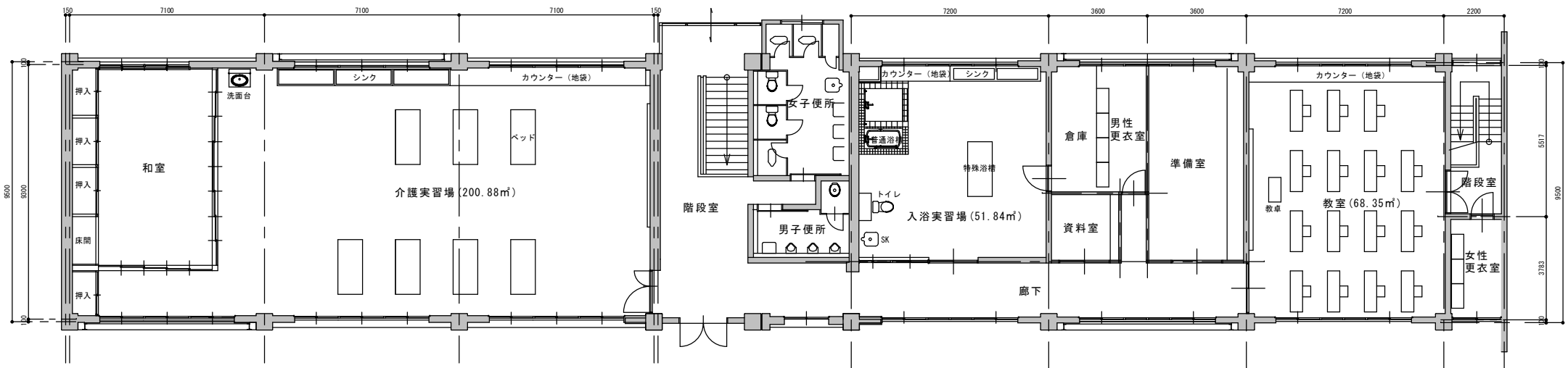
介護サービス科教室・実習室平面図 S=1:100
