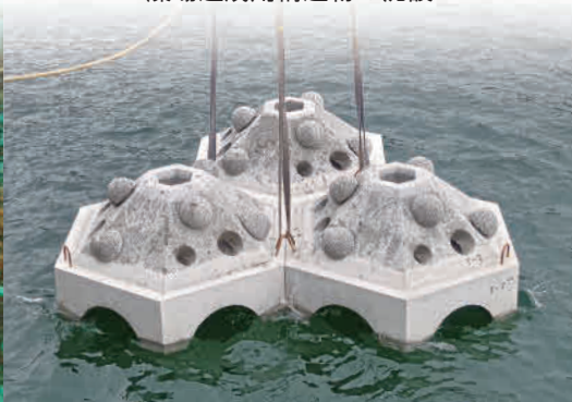
藻場造成用構造物の沈設
