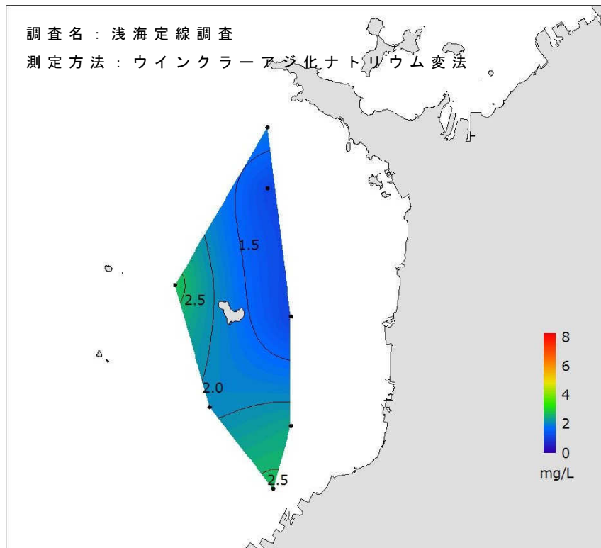
底層の溶存酸素濃度分布
