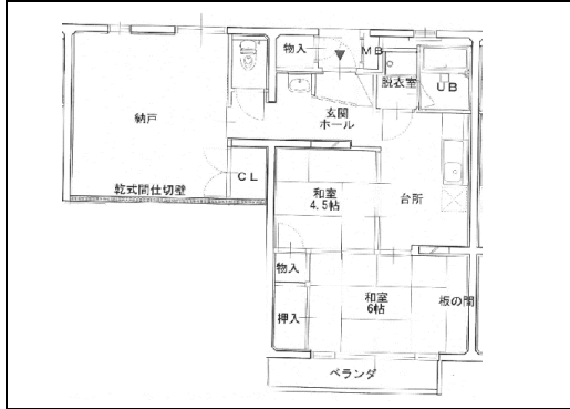
間取例（2UDK）
