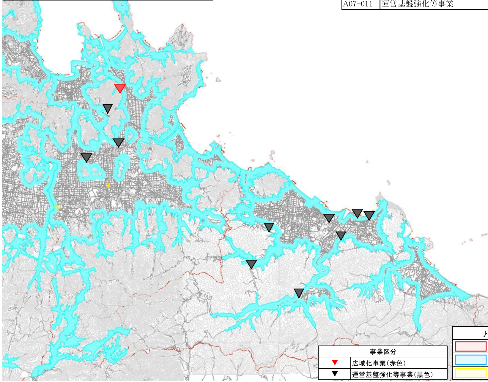
香川県広域水道企業団 水道計画図（東讃地区）
