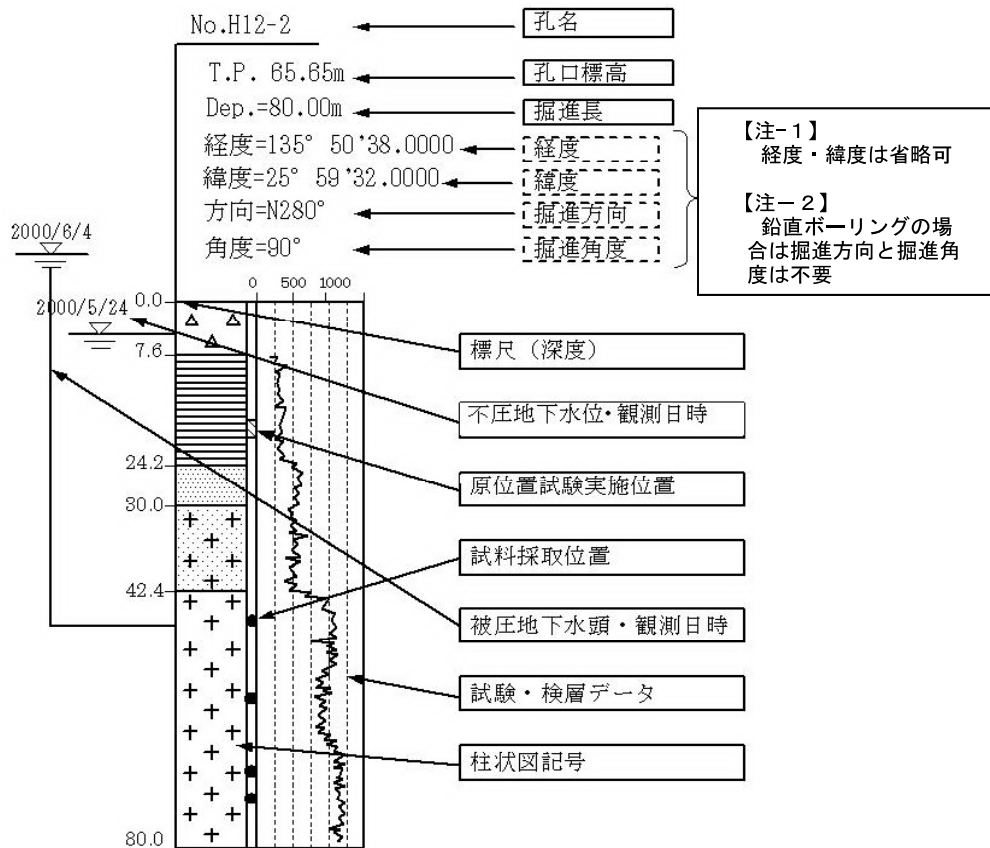
図 3-5 簡略柱状図の記載例 (2 / 2)
