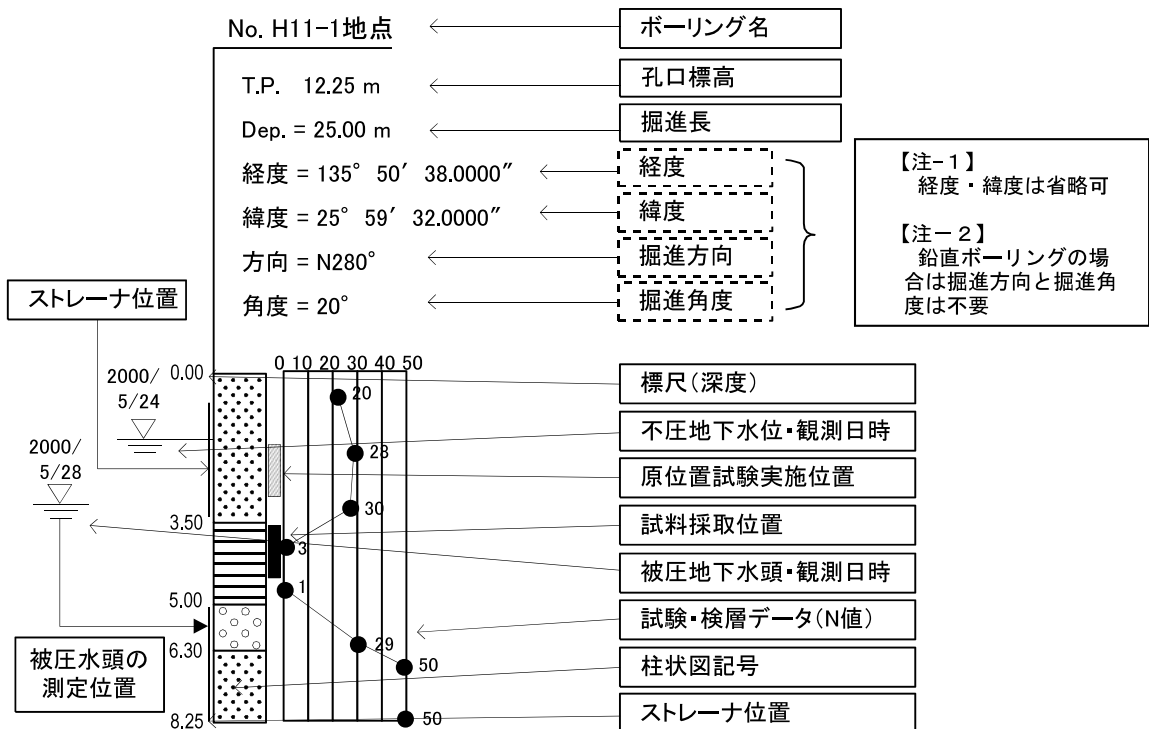
図 3-5 簡略柱状図の記載例 (1/2)
