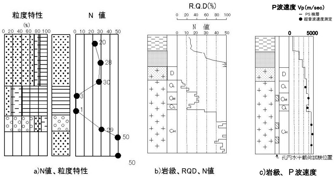
図 3-8 複合表示させた場合の記載例
