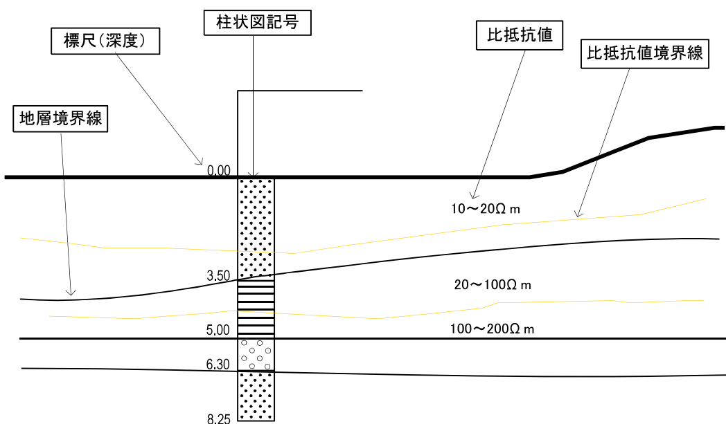
図 3-12 比抵抗断面図の記載例
