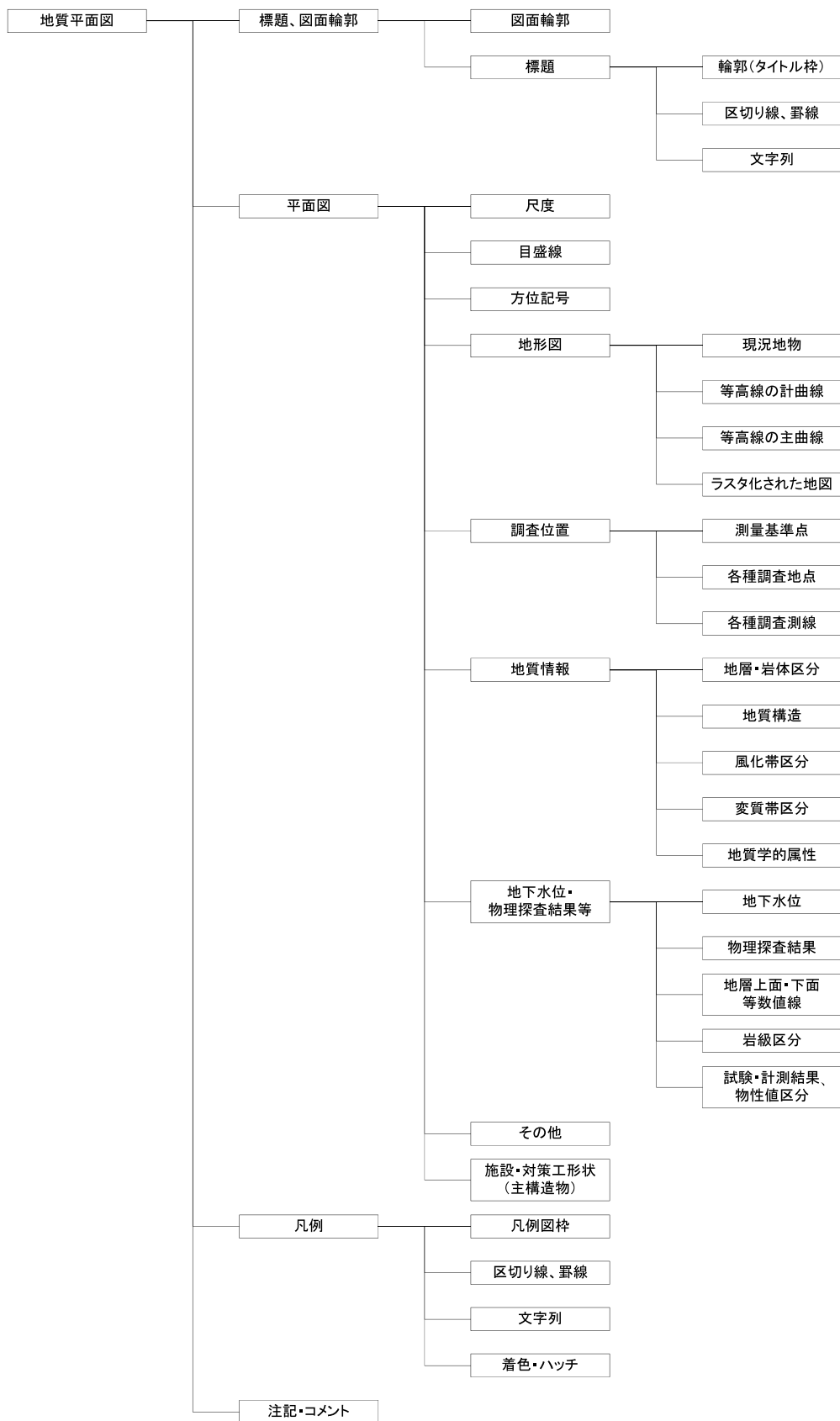
図 3-1 地質平面図の構成要素
