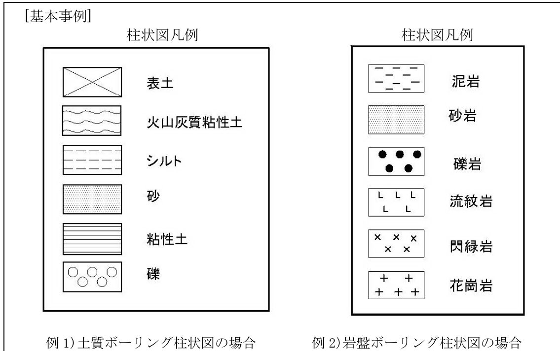
図 3-23 簡易柱状図の凡例の記載例
