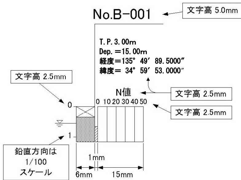
図 7-3 電子簡略柱状図の標準寸法
