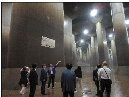
④ 首都圏外郭放水路 (庄和排水機場)
