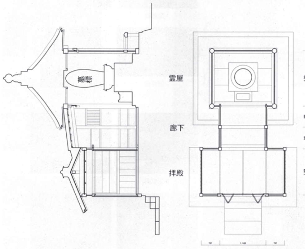
本堯寺松平頼該靈廟平・断面図
