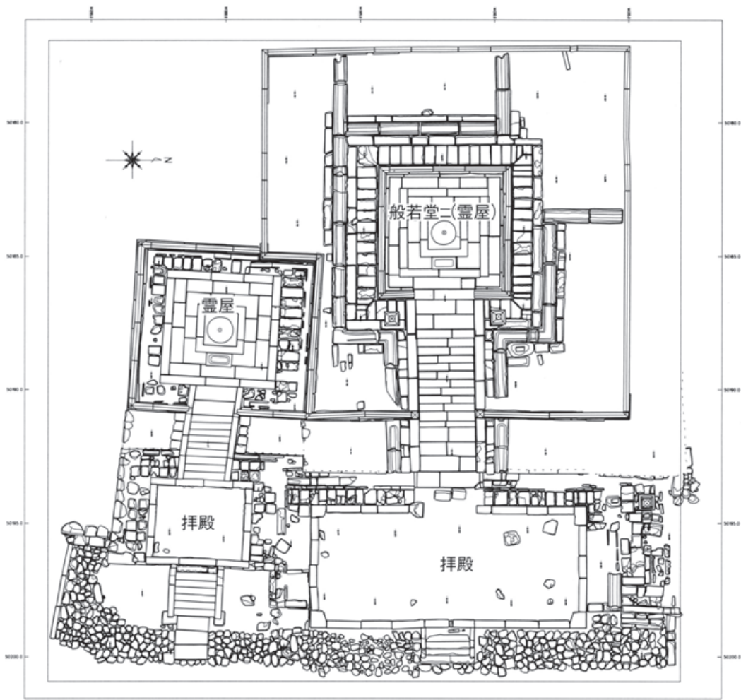
高松松平家法然寺墓所 頼重墓・頼豊墓平面図 (愛媛大学法文学部日本史研究室提供)
