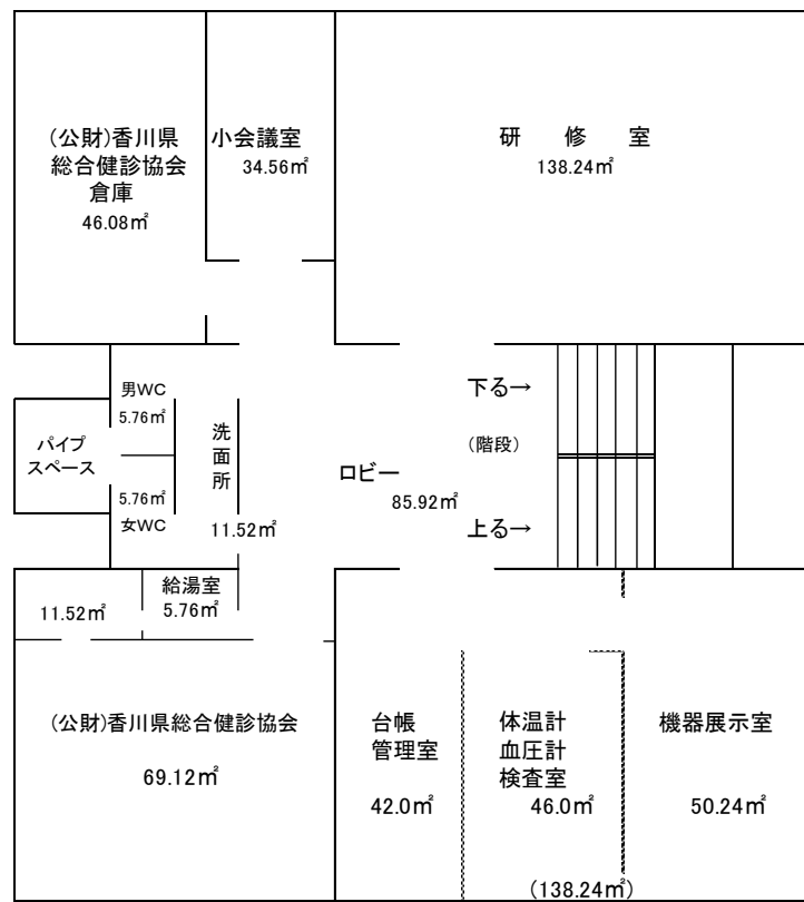
< 2 階平面図 >
