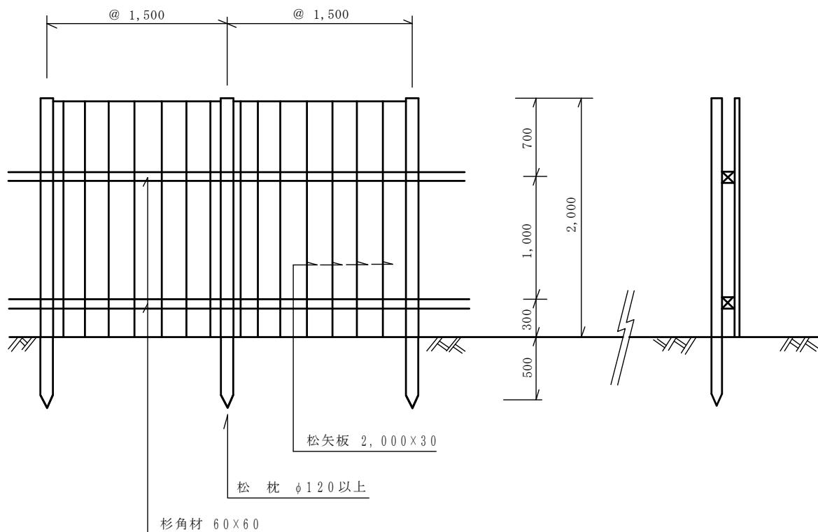
図－2 土留柵図
