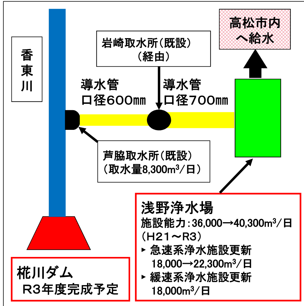
図-2 栴川ダム水運用フロー図(8,300m 3 /日)
