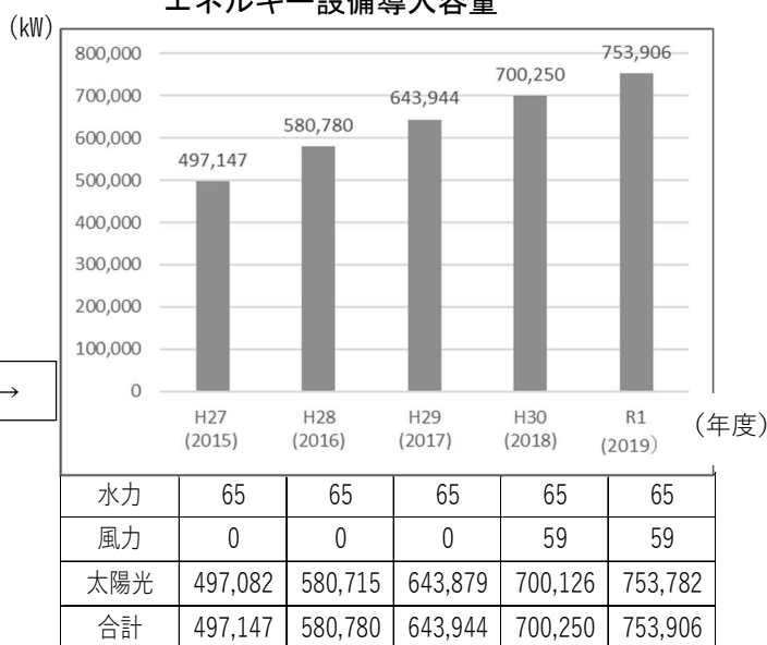
図2-6-4 固定価格買取制度に基づく本県の再生可能エネルギー設備導入容量
