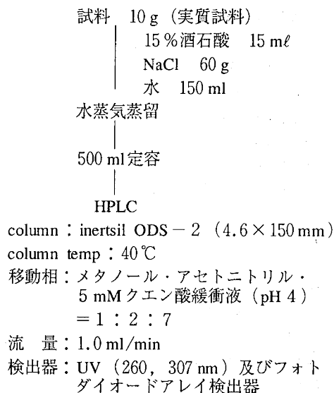
図1 ソルビン酸及びデヒドロ酢酸の分析法
