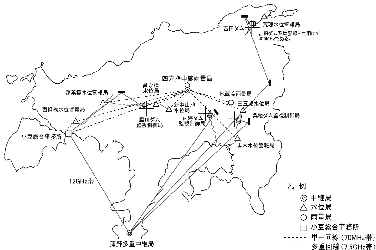
(15) 殿川・内海・栗地・吉田ダム(放流警報)系統図
