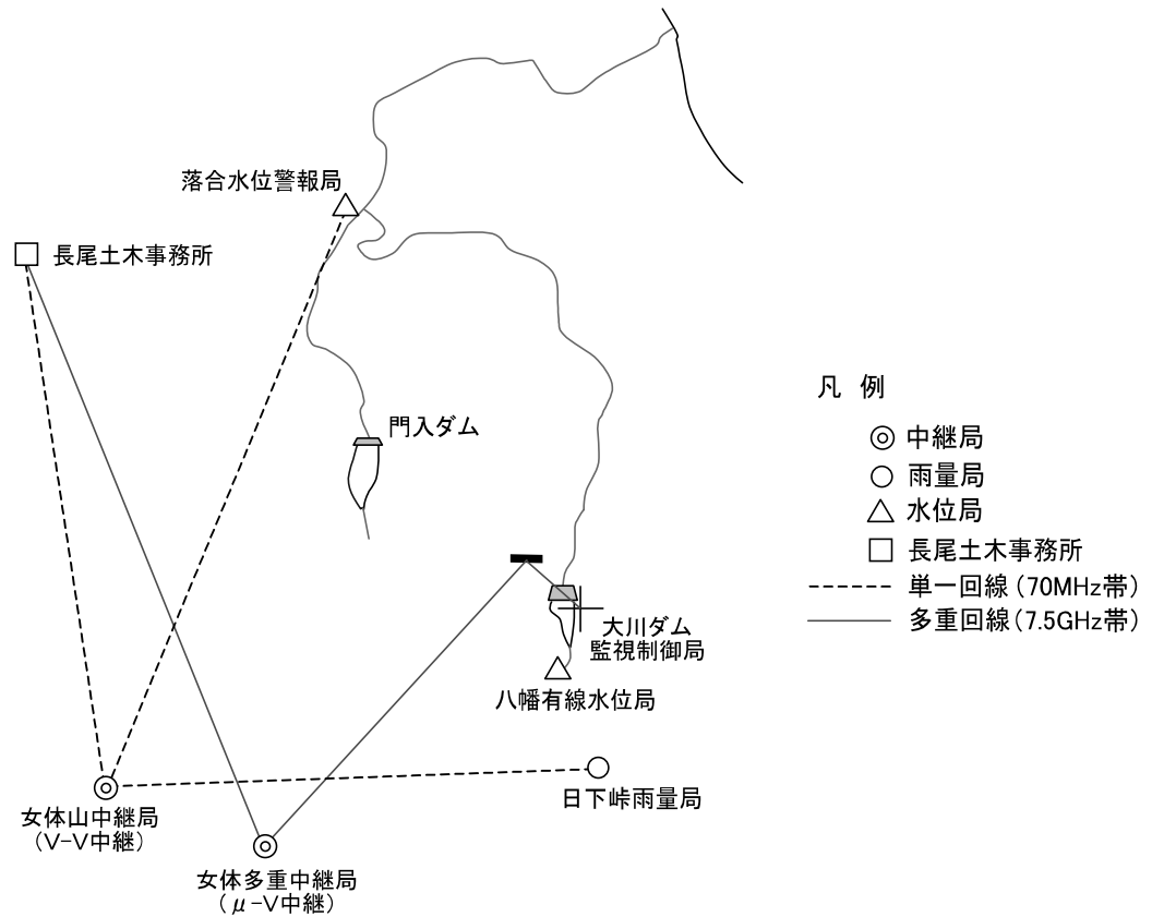
(7) 大川ダム(テレメータ、ダム諸量)系統図
