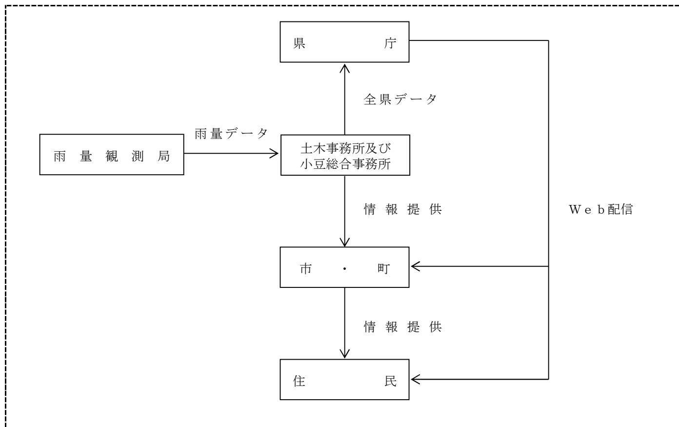
砂 防 情 報 シ ス テ ム 概 要 図
