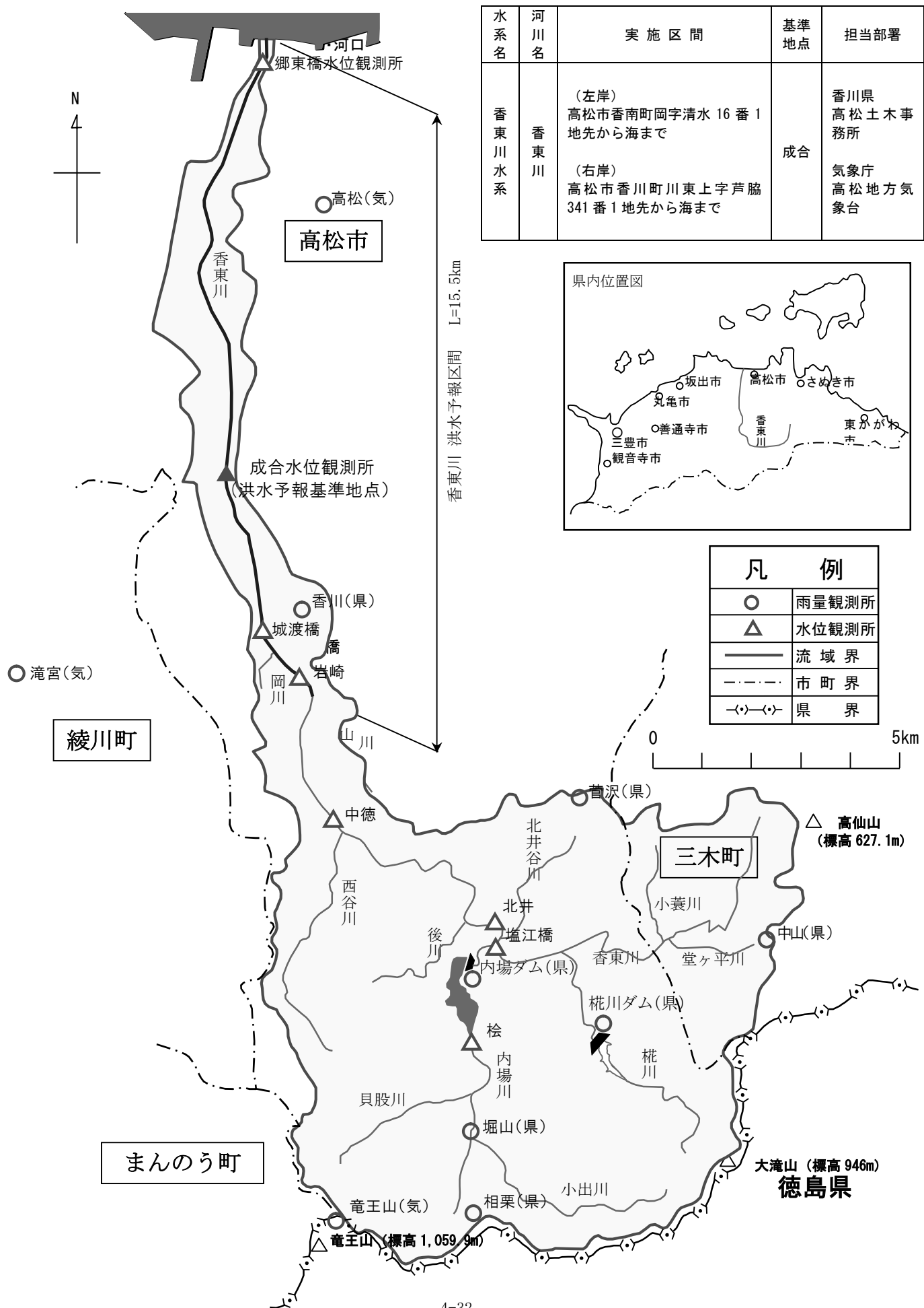
付図1 香東川洪水予報区間及び雨量・水位観測所の位置図
