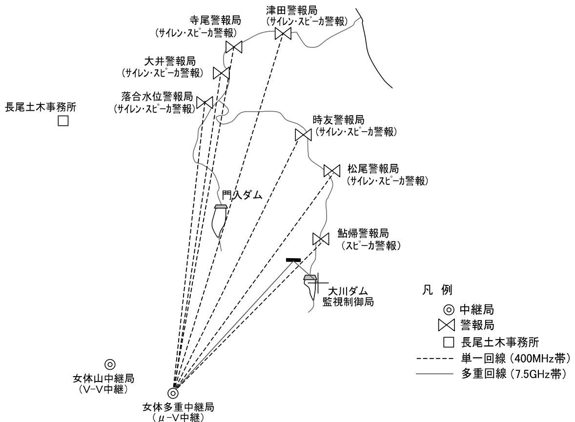
(8) 大川ダム(放流警報)系統図
