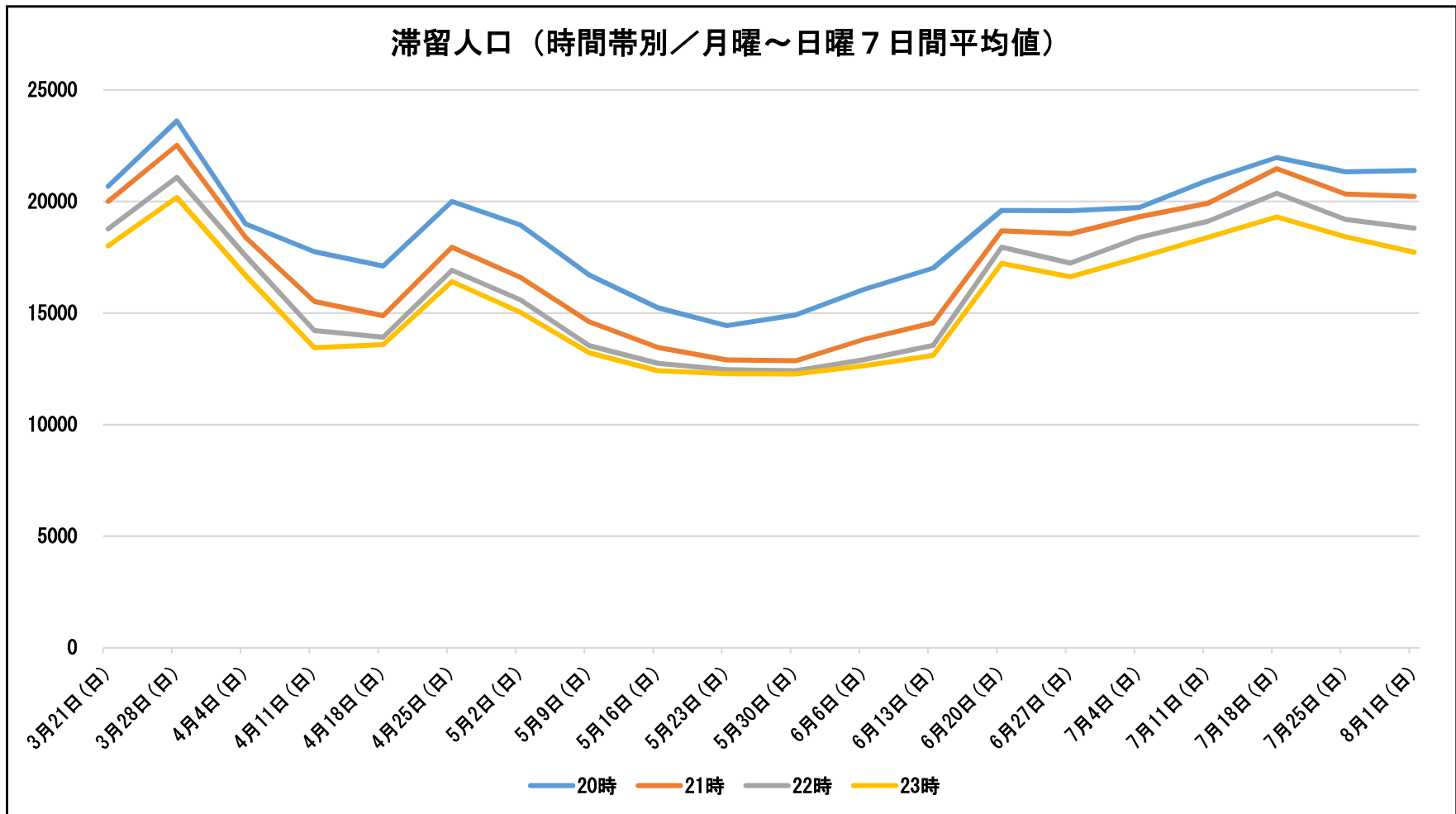
瓦町駅（常磐町商店街、南新町商店街、田町商店街）周辺 500m の滞留人口 出典：Agoop（アグープ）提供データ
