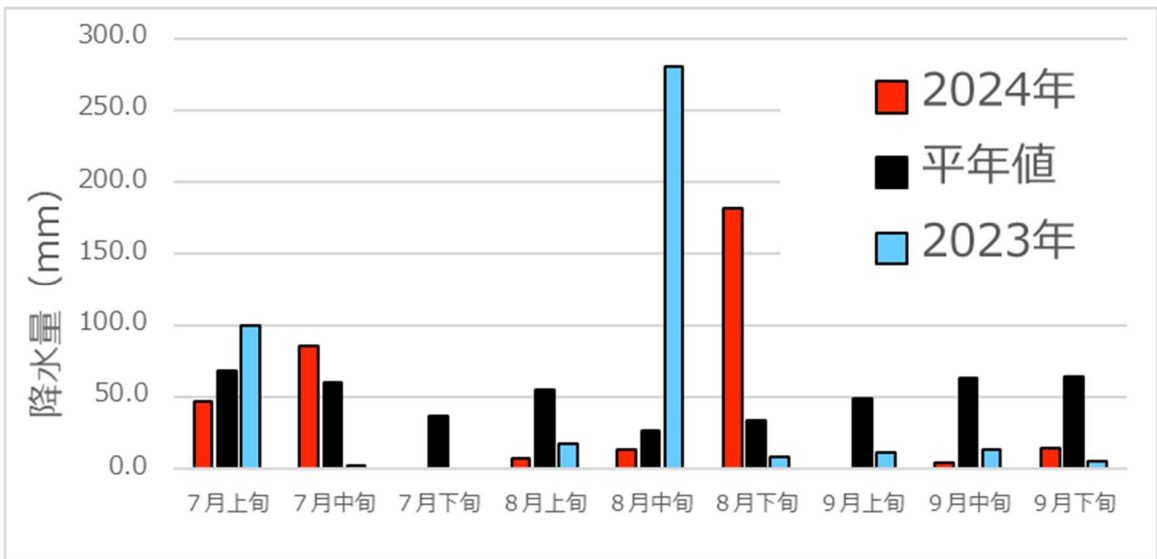
図2 降水量の推移について
