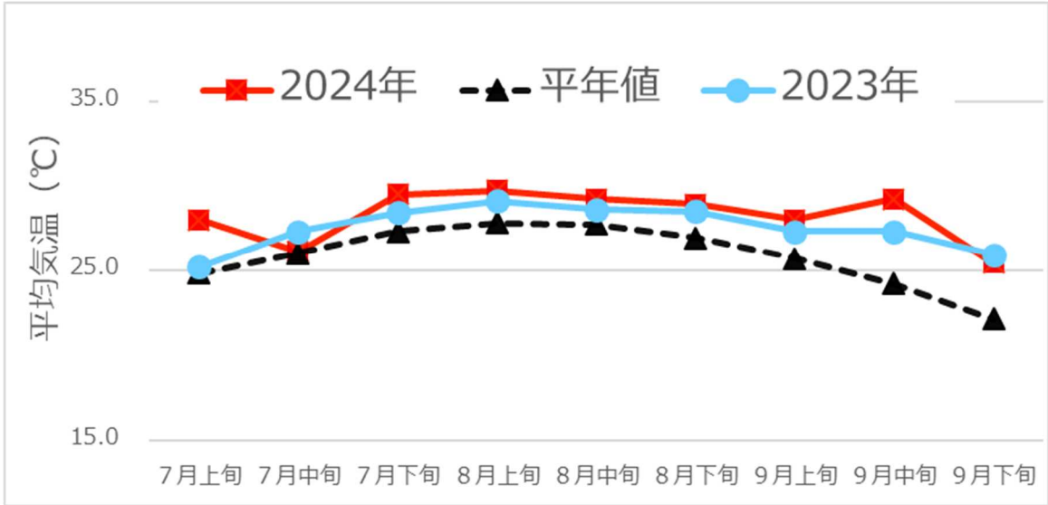
図1 平均気温の推移について
