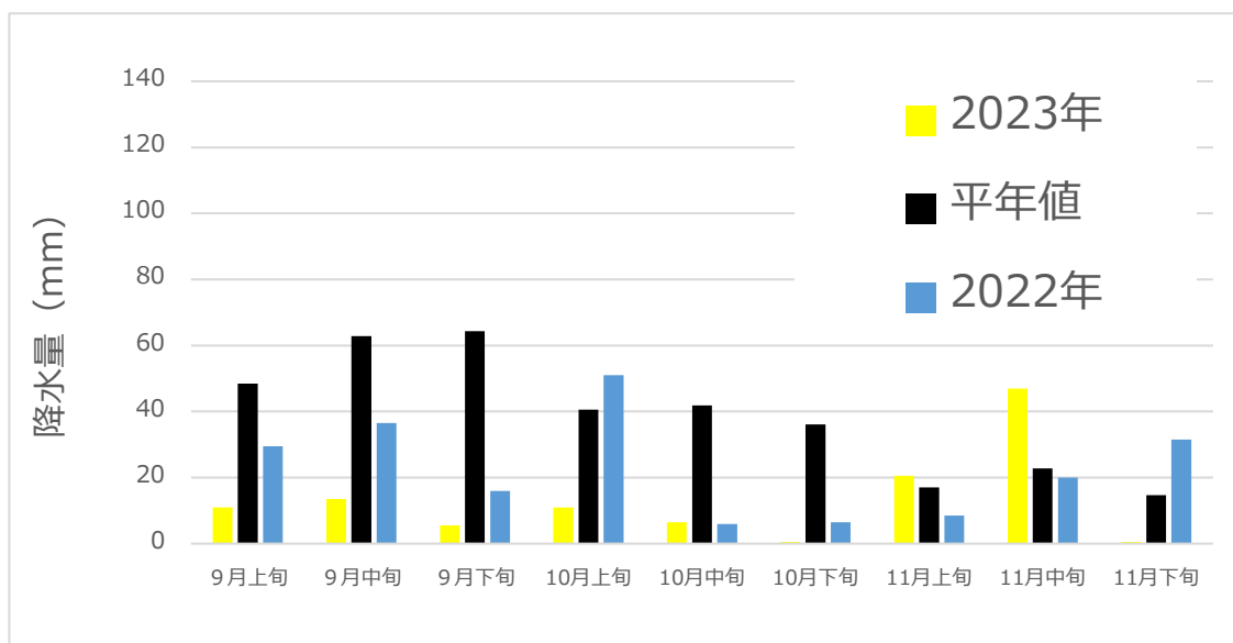
図2 旬別降水量の推移（内海アメダス）
