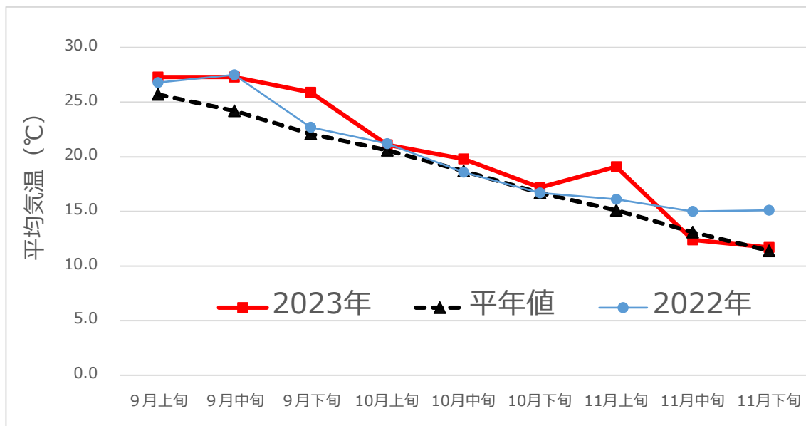
図1 旬別平均気温の推移（内海アメダス）
