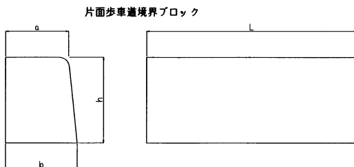
片面歩車道境界ブロック寸法表
