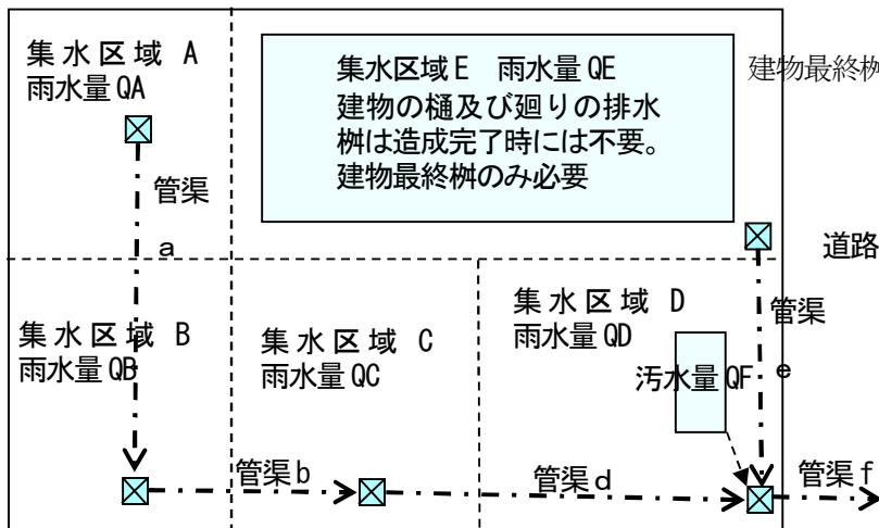
(例2) 予定建築物と屋外とに分けて屋外部分を分割する場合
