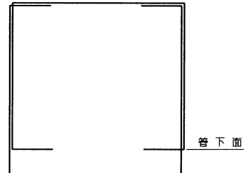
P3型 (D350以下) 鉄筋組立図
