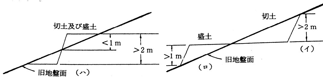
切土又は盛土
