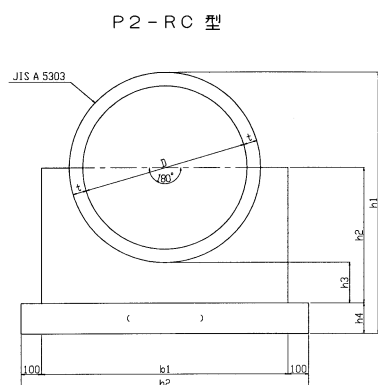
P2-RC型 (パイプカルバート: 180° 固定基礎: 遠心力鉄筋コンクリート管) 寸法および材料表
