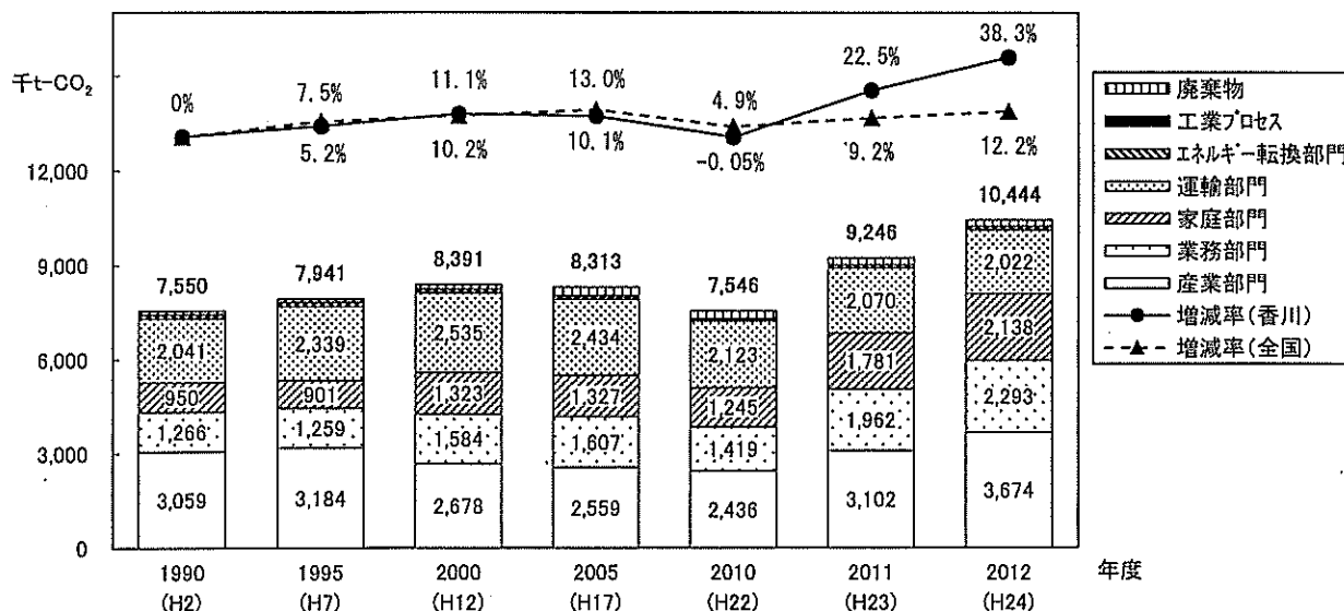
図 3-2-1 CO 2 排出量の推移(部門別)
