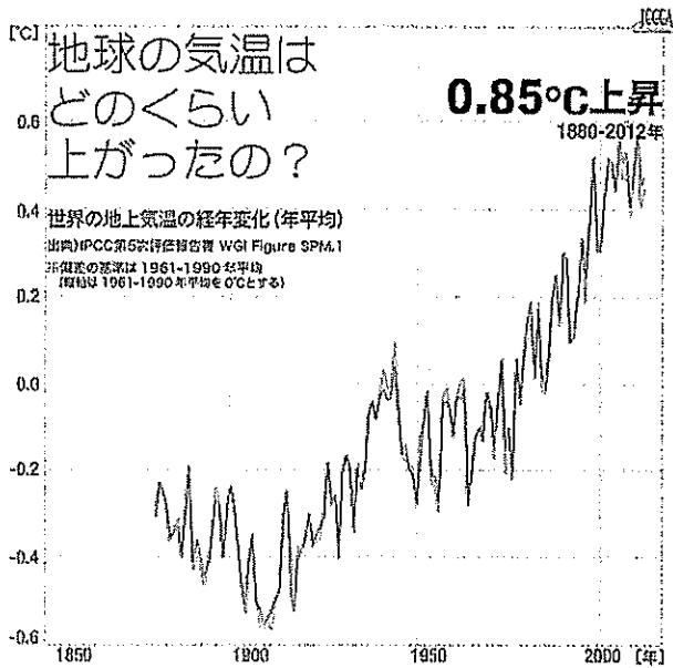
図 1-1-2 地球の気温
