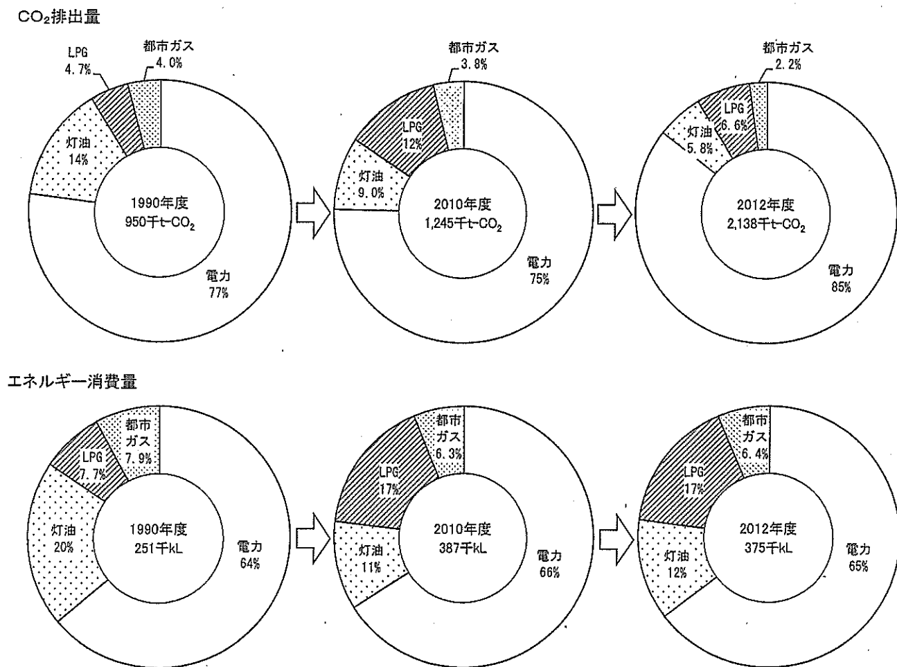
図 3-2-3-6 家庭部門のCO 2 排出量及びエネルギー消費量の構成割合(燃料種別)
