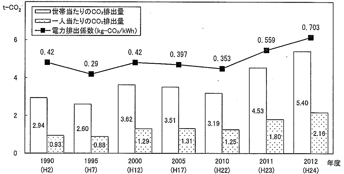
図 3-2-3-4 世帯及び人口当たりのCO 2 排出量の推移
