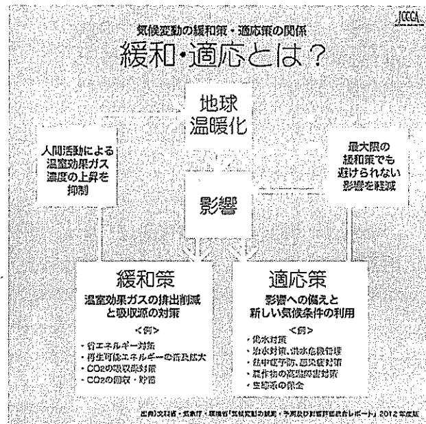
図 1-1-4 緩和・適応
