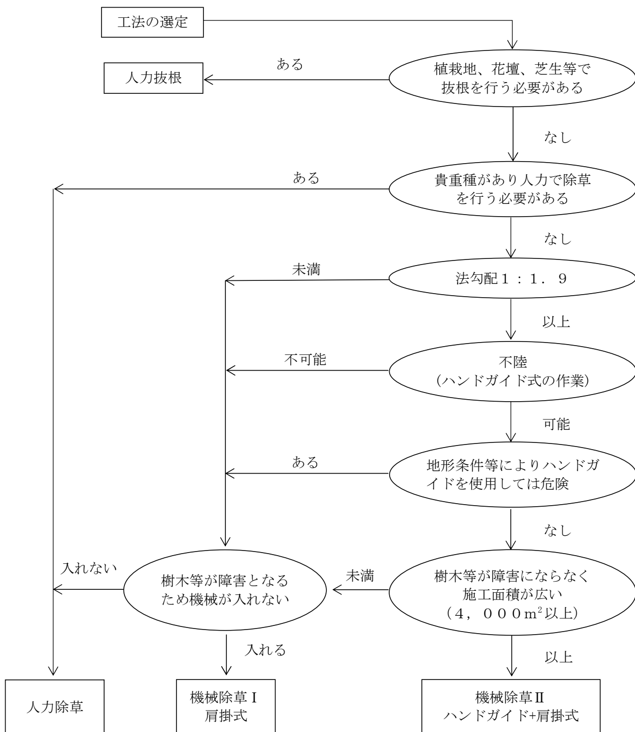
工法の選定フロー
