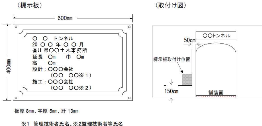
図 6－2 標示板の配置イメージ図
