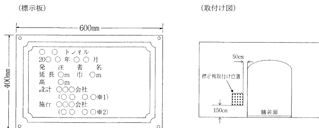
図6-7-2 標示板の刻示標準図
