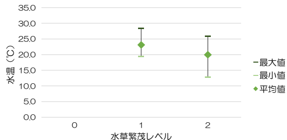
水温：3号堰上流地点（底層）
