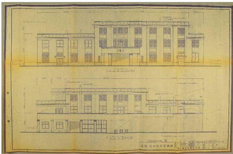
高松港管理事務所改修等工事 添付の建物図 (昭和55年)
