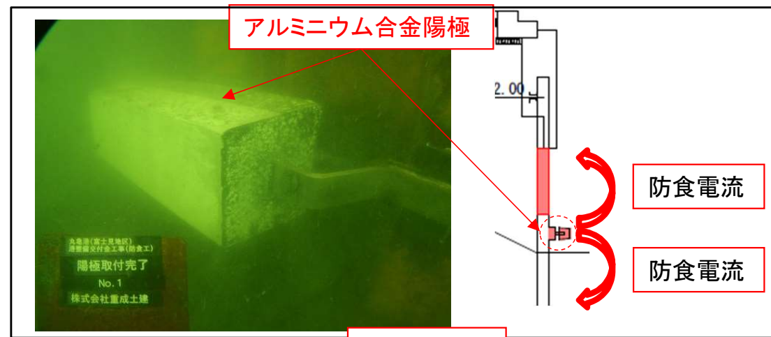
電気防食工
