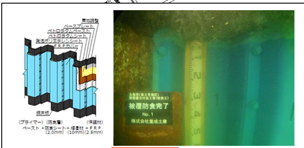
被覆防食工
