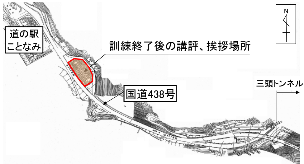
(図三) 香川県側坑口付近平面図
