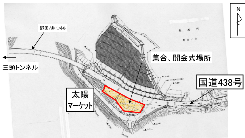
(図一2) 徳島県側 野田ノ井トンネル坑口付近 平面図
