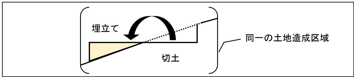
図 4-3 区域内において採取された土砂等を使用して行う特定埋立て等のイメージ
