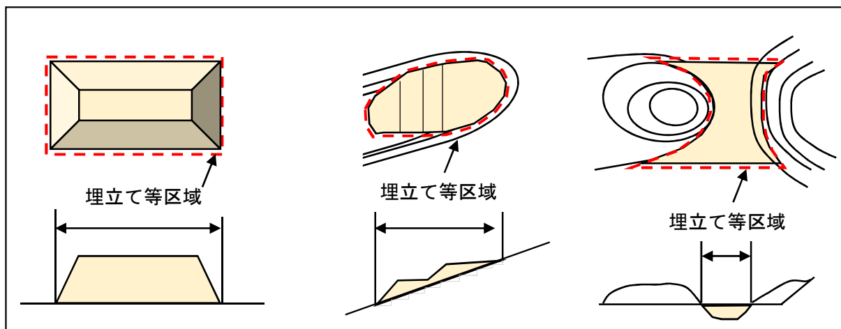
図 2-2 埋立て等区域のイメージ
