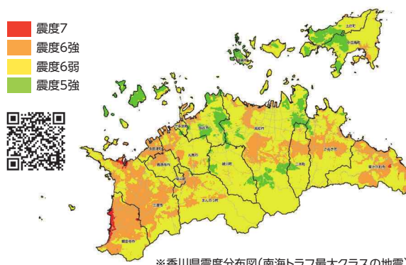
※香川県震度分布図(南海トラフ最大クラスの地震)
