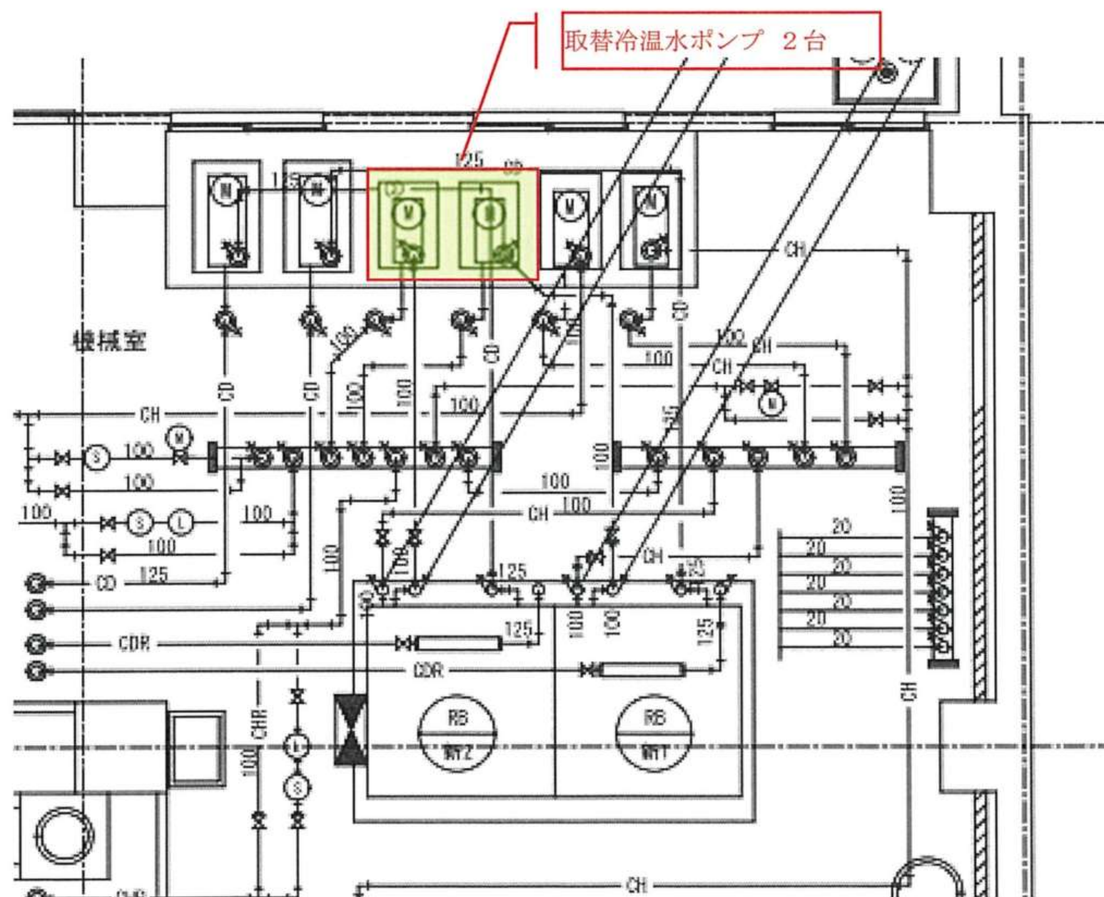
B1F 機械室ポンプ廻り平面図
