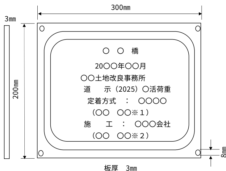
図 12-4-1 橋歴板の記載例
