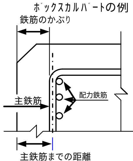
図 3-9-1 鉄筋のかぶり
