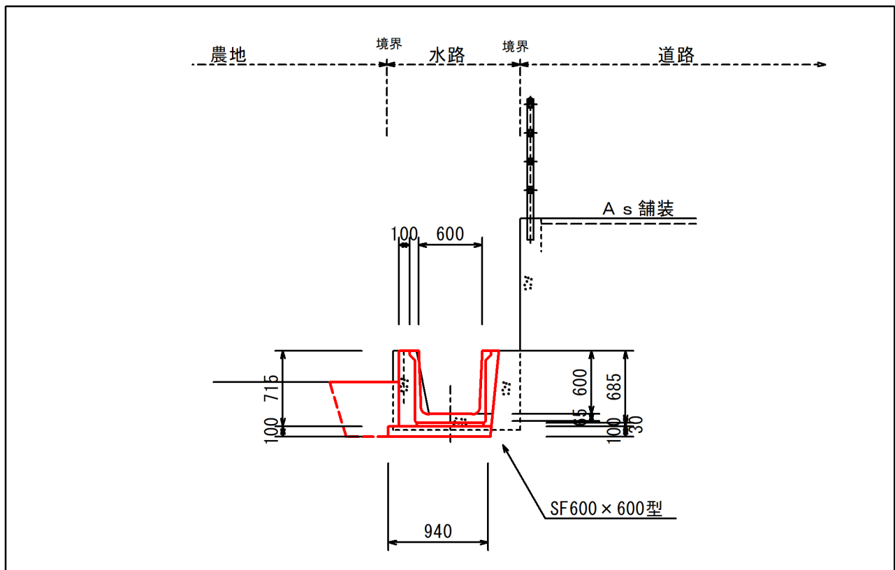
横断面図
